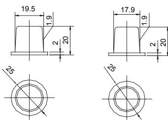
Optional Terminal (SAE)
